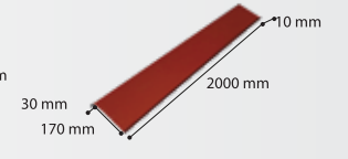
Eco Alın Levhası Profili Eco Forehead Plate Profile
