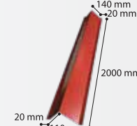
Eco Kar Tutucu Profili Eco Snow Catcher Profile
