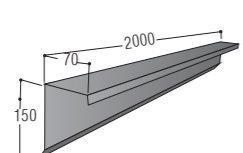
قطعة حافة الهامش الجانبي / Barge Board Flashing
