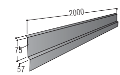
قطعة الجزء السفلي للجدار / Wall Side Flashing
