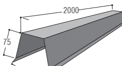
قطعة حافة الرأس / Square Ridge Cape
