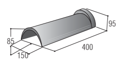
حافة دائرية / Circular Ridge Cape
