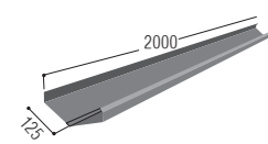
قطعة تركيبية الوادي / Combination Valley
