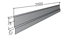
پروفیل گوشه دیوار / Wall Side Flashing
