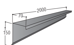
فلاشینگ خط الراهی جانبی / Barge Board Flashing
