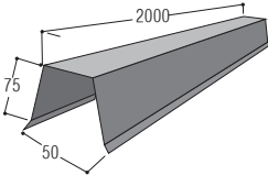
فلاشینگ خط الراس مربعی / Square Ridge Cape
